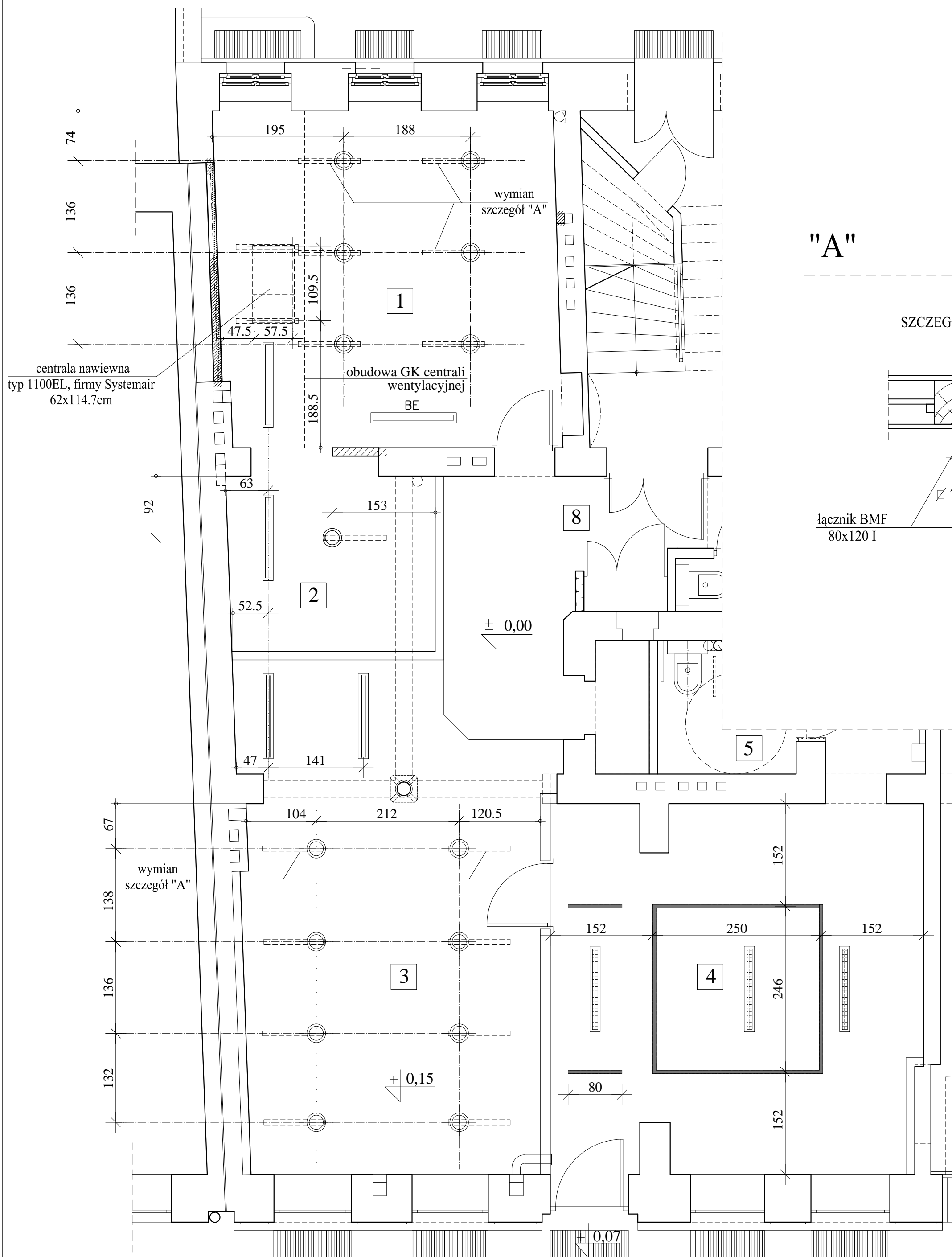
WZMOCNIENIA STROPU POD URZĄDZENIA, ROZMIESZCZENIE ELEMENTÓW OŚWIETLENIA 1:50
